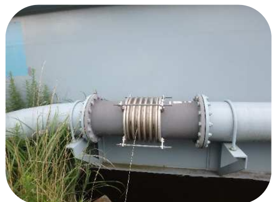
北側道橋添架管(左:補修前、右:補修後)
