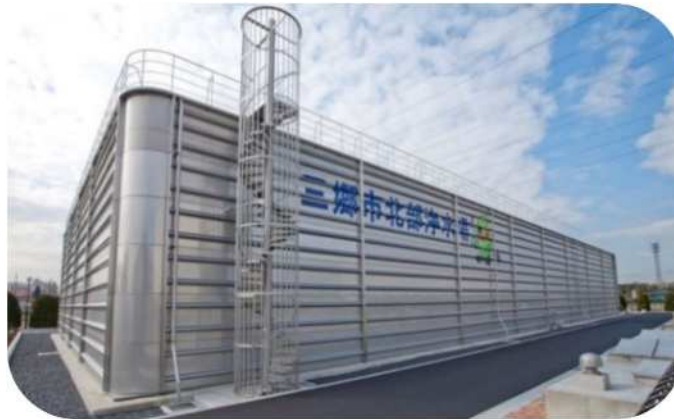
北部浄水場(耐震性ステンレス製配水池)
