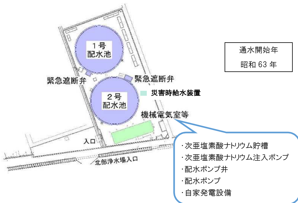
図 2-10. 北部第二配水場の配置図
