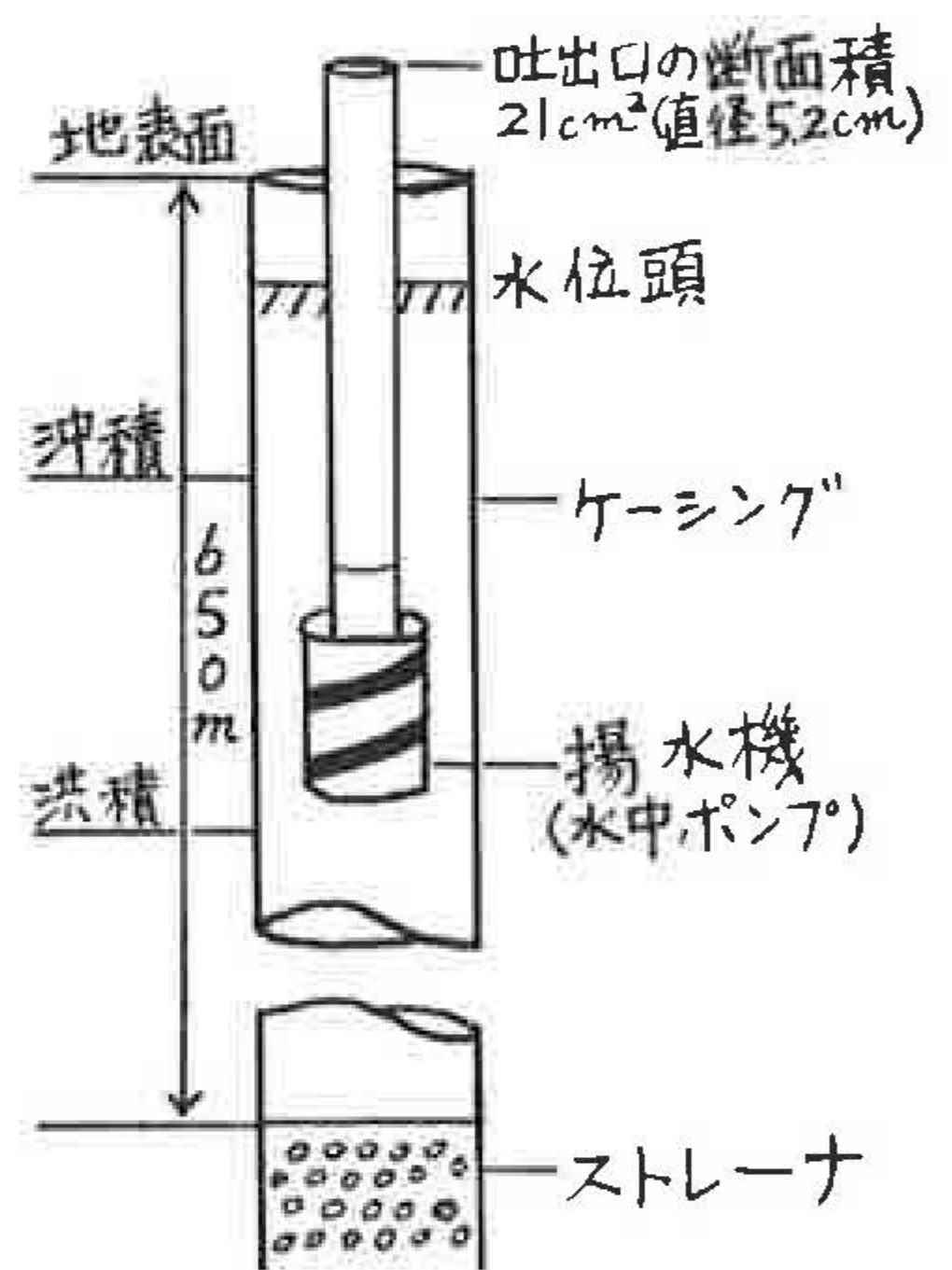
揚水施設構造図
