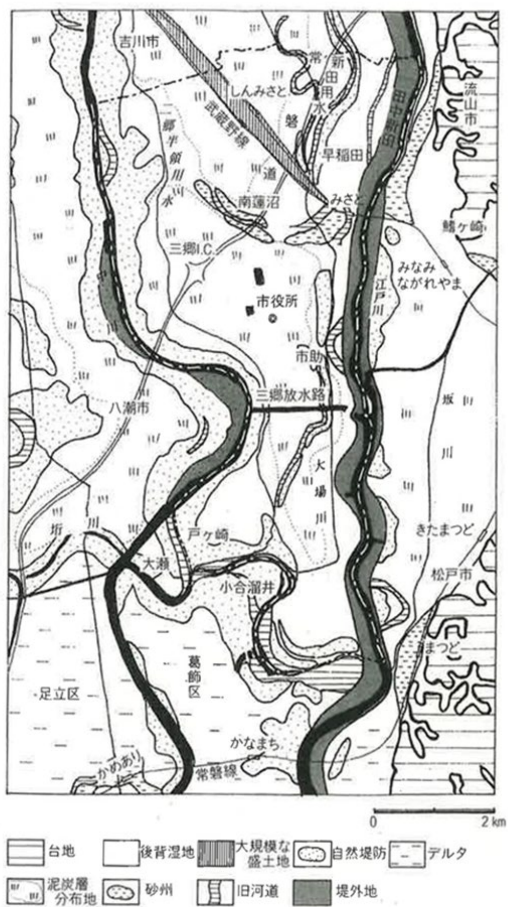
三郷市とその周辺の地形分類図
