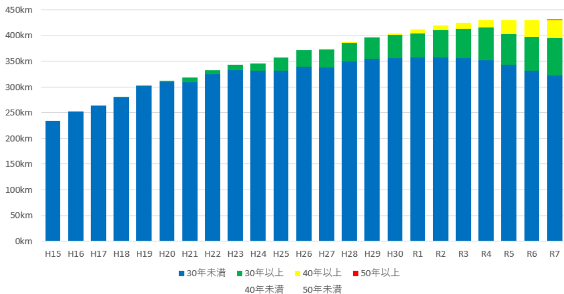
図 1-3 施工経過年数別管渠延長
