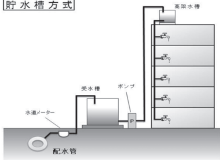
貯水槽方式
