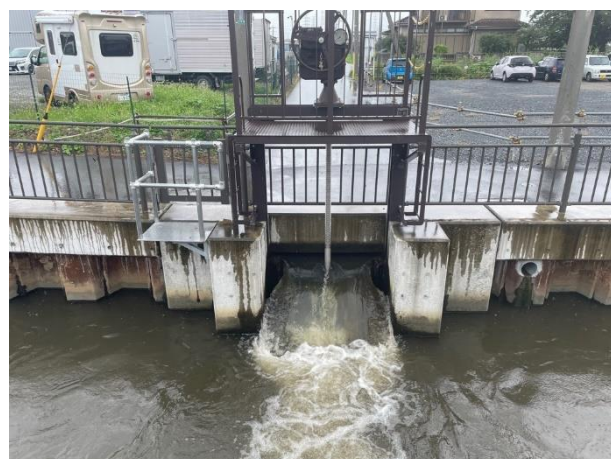
二段式スライドゲート (開度 40 パーセント)
